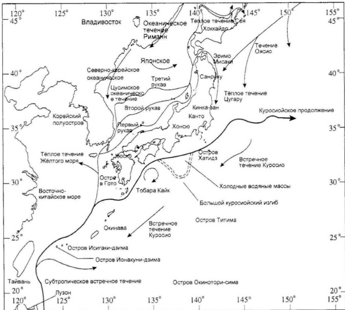
Рис. 1-10. Основные океанические течения в японских водах.
